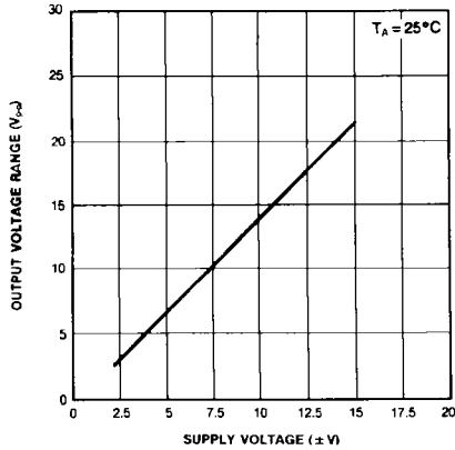
Fig. 3 OUTPUT SWING
